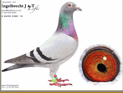
BEST-SHORTCUT
